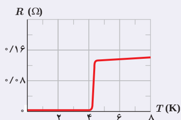
مقاومت ویژه جیوه در دمای حدود 4K به صفر می‌رسد.
