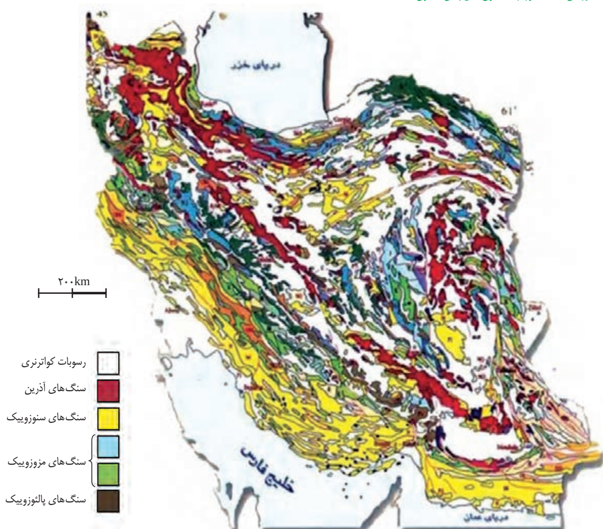
شکل ۷-۶. نقشه زمین‌شناسی ایران که نشان‌دهنده پراکندگی سنگ‌های زمان‌های مختلف زمین‌شناسی با رنگ‌های متفاوت می‌باشد.
