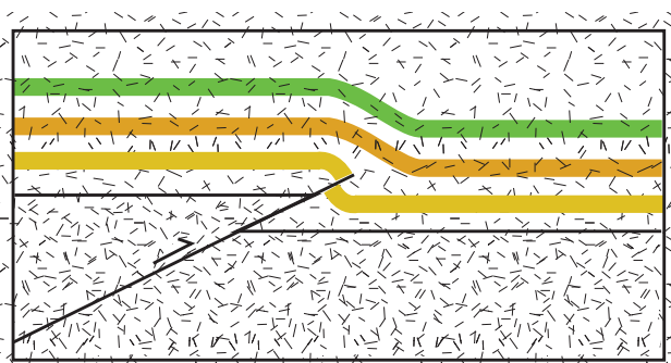
(الف) گسل معکوس
