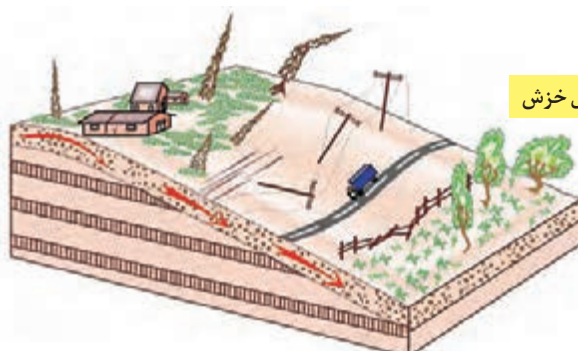
حرکت کند و نامحسوس رسوبات سطح دامنه در مدت زمان طولانی
