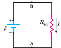
شکل ۲۰-۲ مدار معادل شکل ۱۹-۲ جریان آنها داریم: که در آن سه مقاومت با مقاومت R_{eq} جایگزین شده است. و در نتیجه
