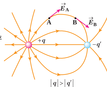
شکل ۱۷-۱ خطوط میدان از بارهای مثبت
